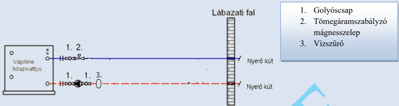
13.ábra Aktív hűtésű hőszivattyú kút oldali bekötése
