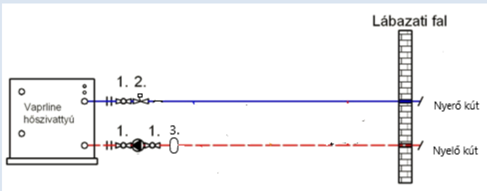
13.ábra Aktív hűtésű hőszivattyú kút oldali bekötése
