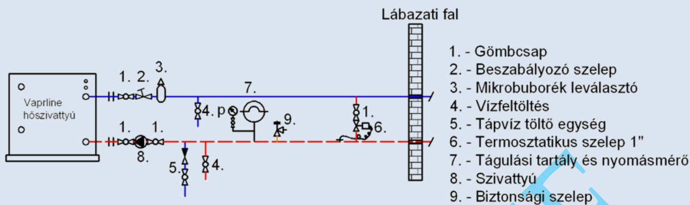
13.ábra Aktív hűtésű hőszivattyú föld oldali bekötése, passzív hűtés nélkül
