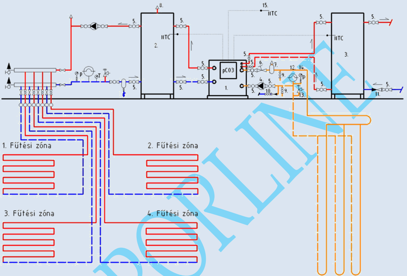
12.ábra Hőszivattyús hőközpont kapcsolási sémája
